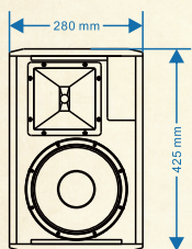
主视图
